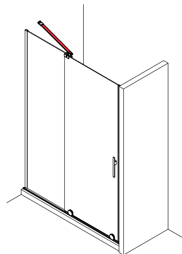
Solution de façade entre 2 murs avec tendeur sur mur latéral (Page 500)+ kit de fermeture magnétique en option
