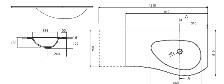
Plan vasque MAM 1200 coquette à gauche Charge minérale blanc brillant sans siphon ni bonde de vidage clic- clac ni mitigeur 1210 x 16 x 510 mm 85906 269 €
