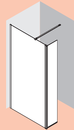
PAROI 1 FIXE + 1 VOLET PIVOTANT
