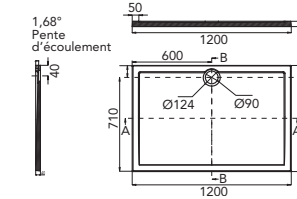
RECTANGLE 120 X 80 CM BONDE CENTRÉE Garantie 5 ans
